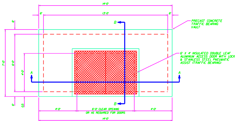
TOP PLAN SCALE: 1/2" = 1'-0"
